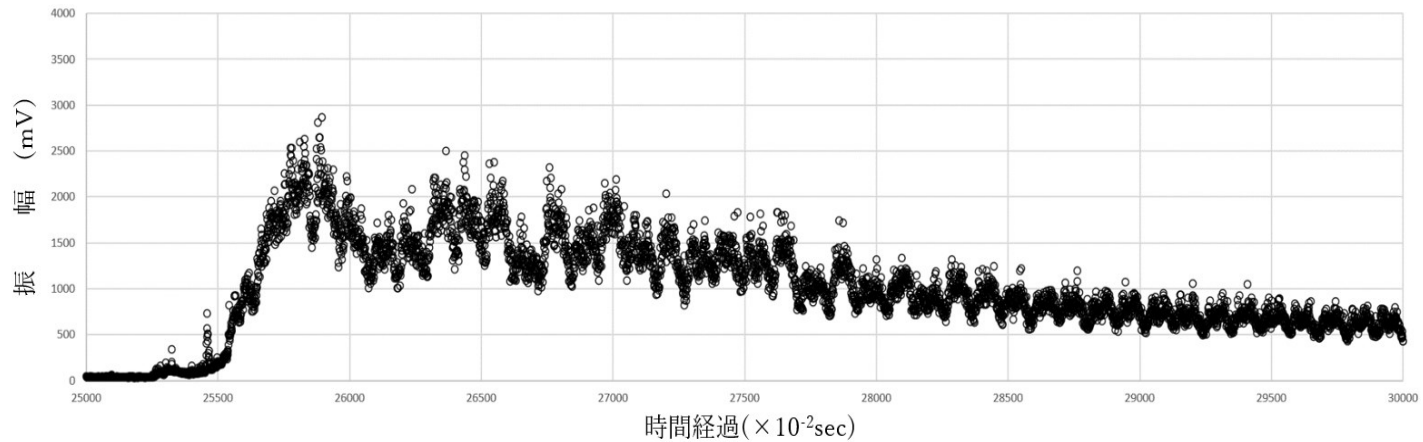
ハンバーグ原料混合過程におけるAEの挙動
